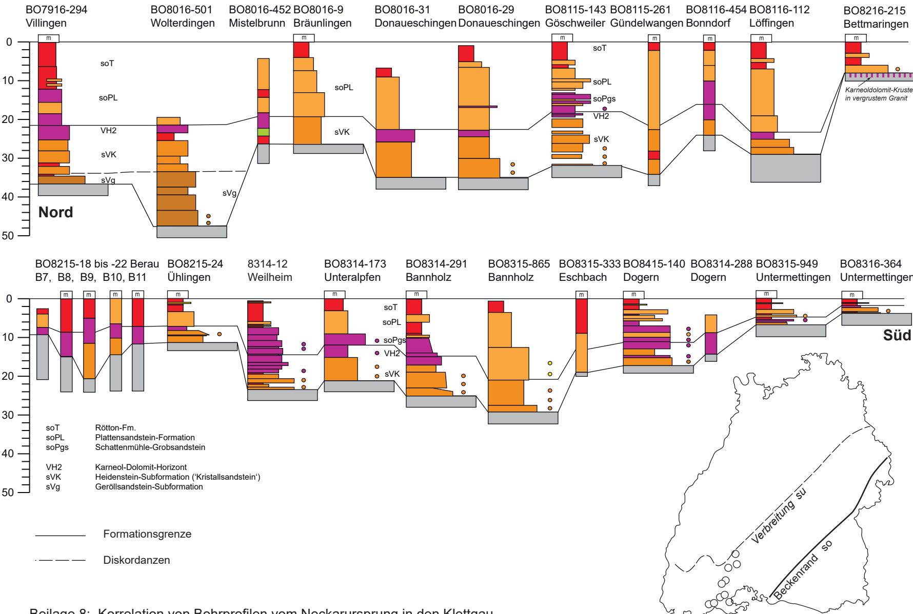
Beilage 8: Korrelation von Bohrprofilen vom Neckarursprung in den Klettgau
