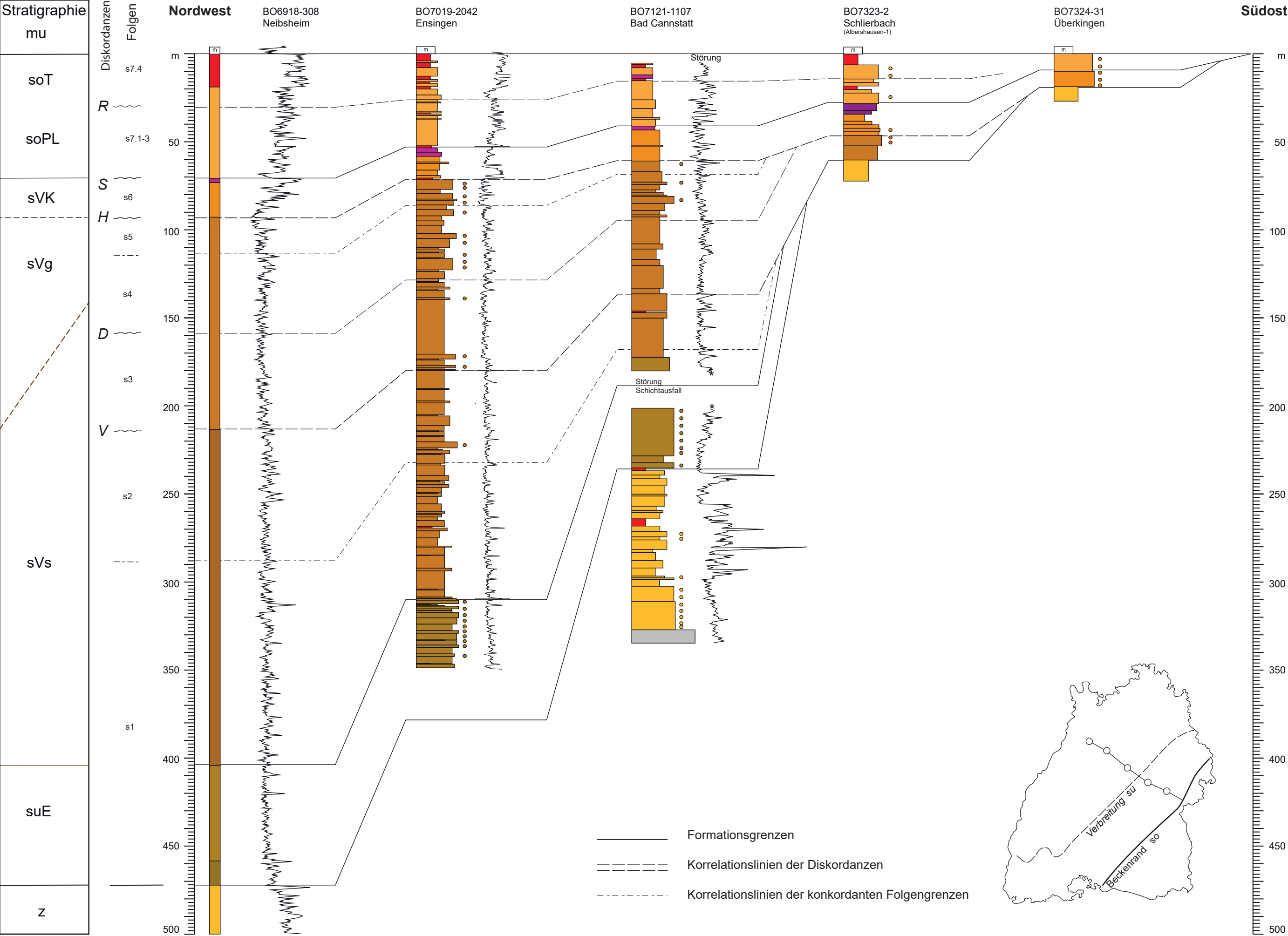
Beilage 1: Zusammenfassende Übersicht der Korrelationsergebnisse anhand eines NW–SE-Profiles
